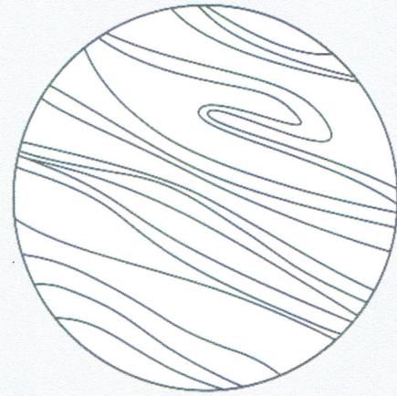
Jowisz
