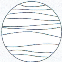
Wenus
