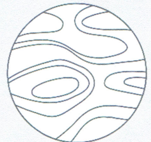
Neptun
