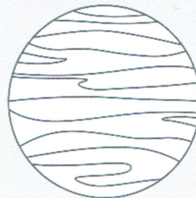
Uran
